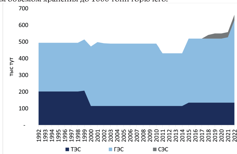
Рис. 7. Установленная мощность афганских электростанций, 1992–2022 гг.
